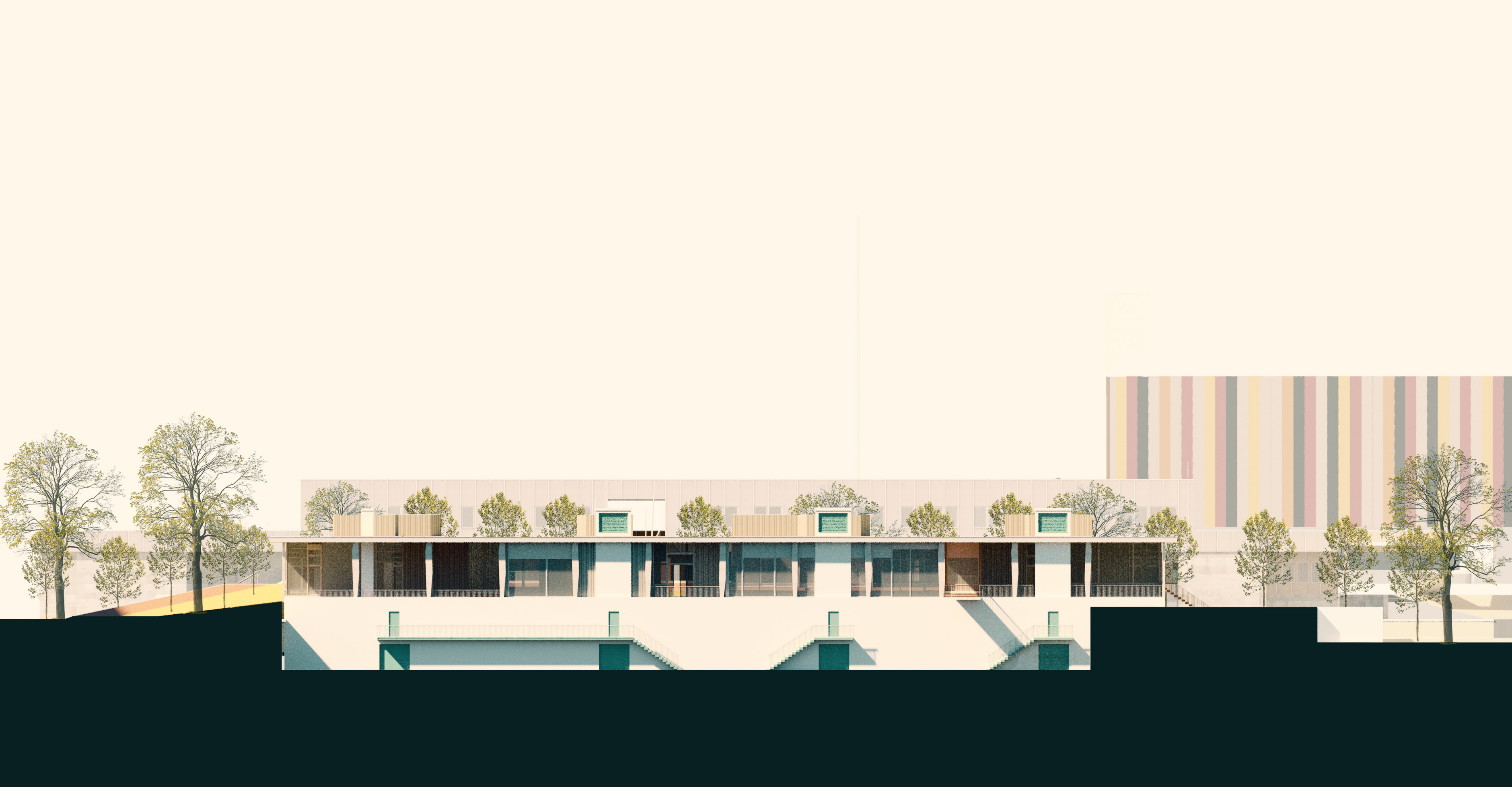
POHLED ZÁPADNÍ 1:250
