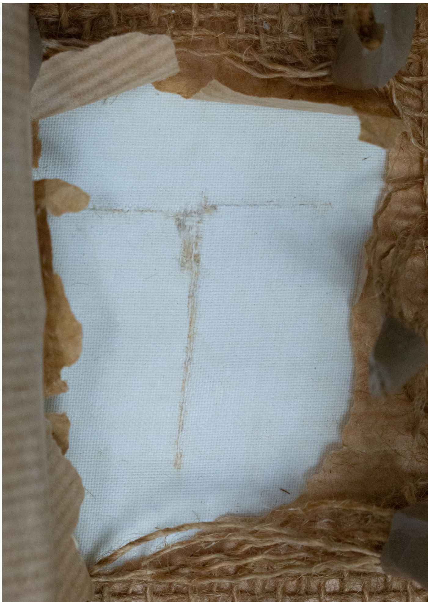
Dokončení scelování jemného bavlněného plátna polyamidovým práškem a tepelnou špachtlí metodou vlákn no na vlákno
